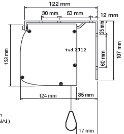
Gehäuse Abmessungen
